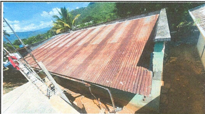
Foto1: Cambio de lámina troquelada calibre 26, con lijado y pintado de la estructura metálica de techo existente, e instalación de canal metálico con bajadas pluviales en tubo PVC de 3" color blanco.
