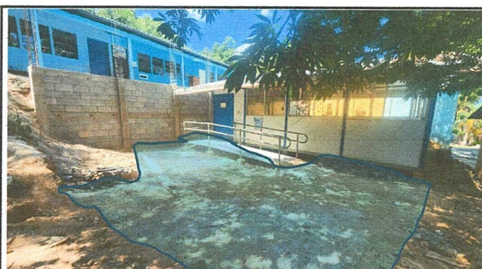
Foto 4: Colocación de torta de concreto de 7 cm de espesor, con un área total de 40 m².
